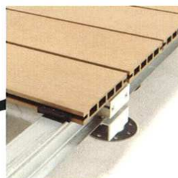
幕板取付け金物
