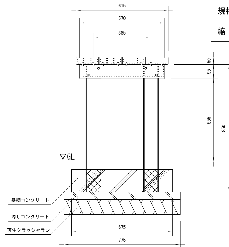
側面図
